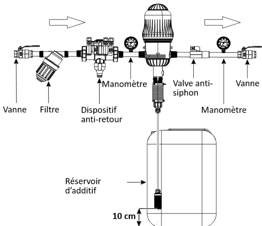
Installation incorrecte
