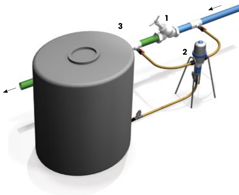
一个典型的旁路安装
