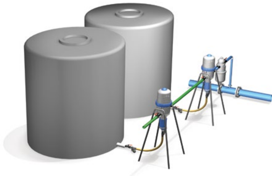
MixRite TF比例混合泵的典型双泵串联安装
